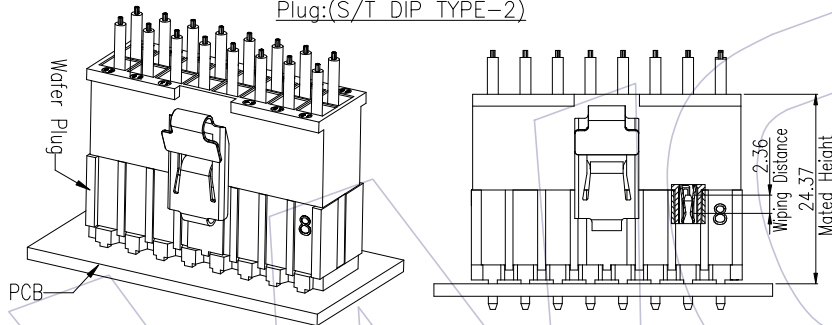
Plug:(S/T DIP TYPE-2)
